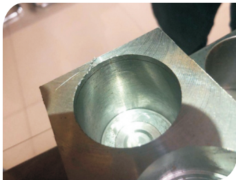
⬆ 未加裝減振機構 ( Ra > 3.2 )
